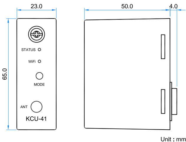
圖一 尺寸圖
